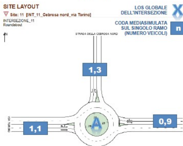
Fig. 3 – intersezione 11: STATO ATTUALE - LOS Globale e lunghezza media simulata delle code
